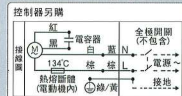
接線示意圖
