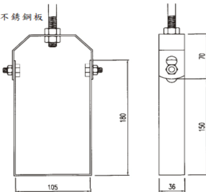
燈用線槽門型吊架
