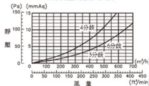
給氣壓力損失曲線
