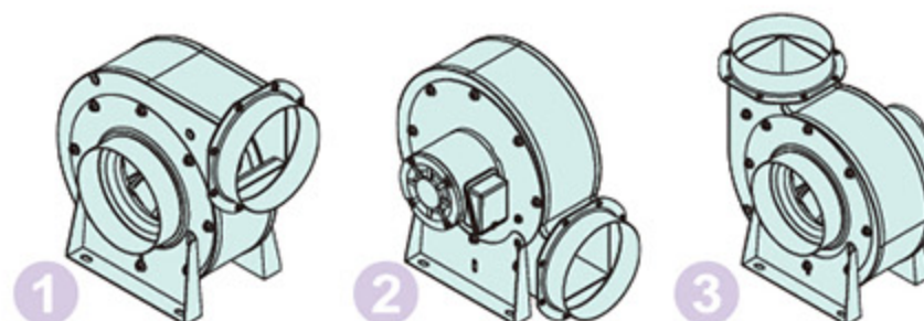
腳座三種方向安裝
