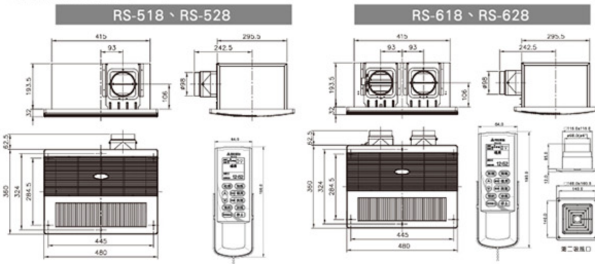
●產品尺寸圖 (單位：mm)
