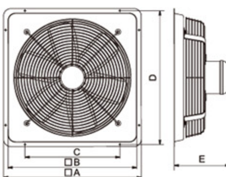
●產品尺寸圖 (單位：mm)
