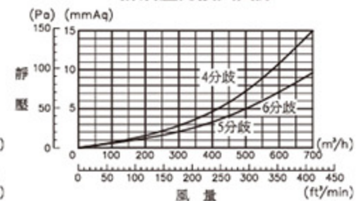
排氣壓力損失曲線
