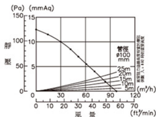
●性能曲線表
