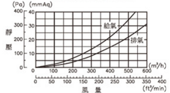
AO-62S 壓力損失曲線
