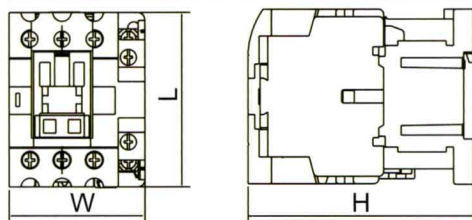
非可逆式電磁接觸器
