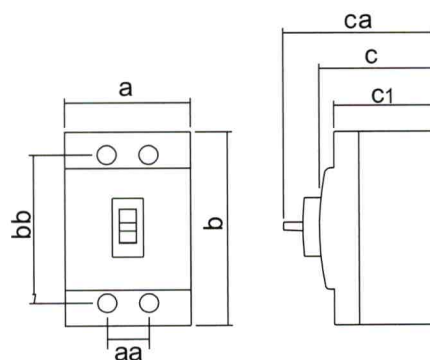
掀蓋式無熔線斷路器
