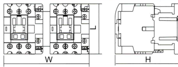
可逆式電磁接觸器
