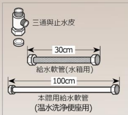
• 配管用零件
